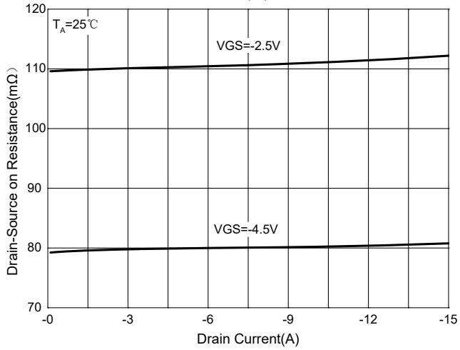
Fig. 7 - R_{DS(ON)} - I_D
