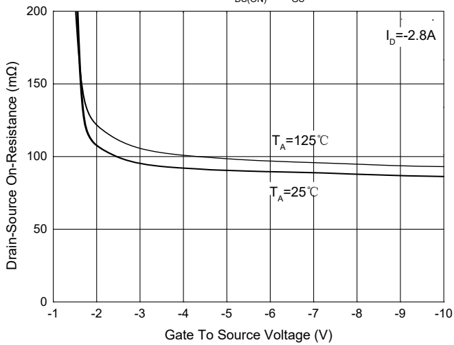
Fig. 9 - R_{DS(ON)} - V_{GS}
