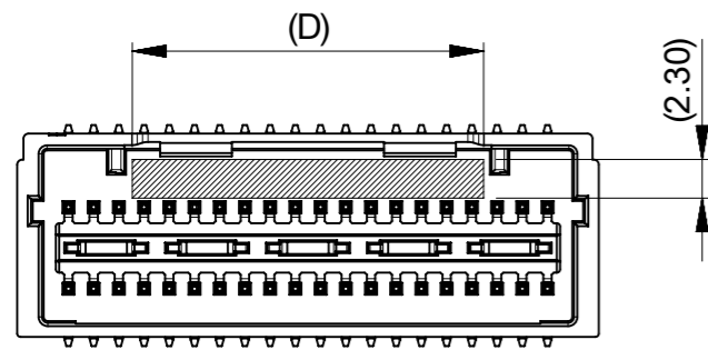
吸着範囲 VACCUME AREA
