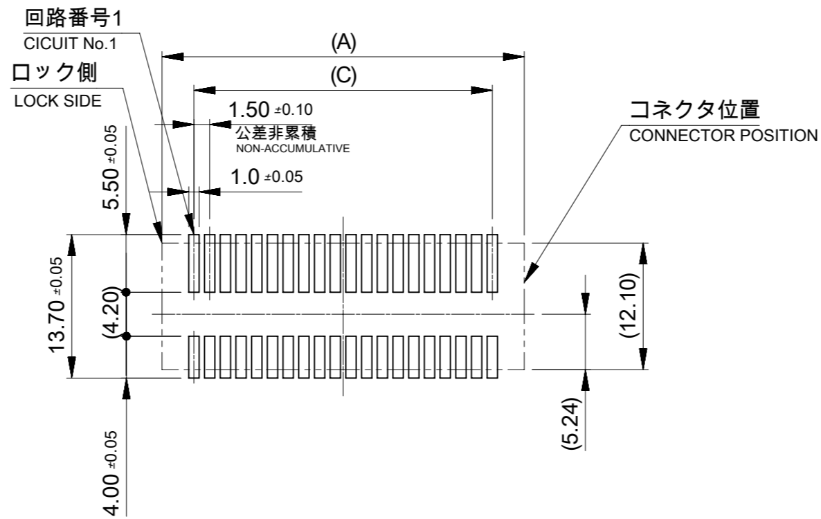
推奨基板パターンレイアウト RECCOMENDED PCB PATTERN LAYOUT
