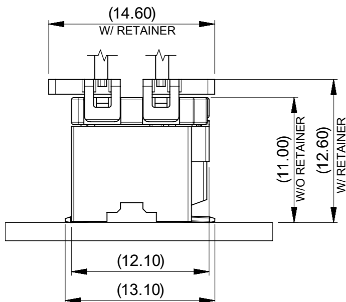
嵌合高さ MATING HEIGHT
