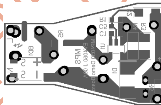
Bottom Layer
