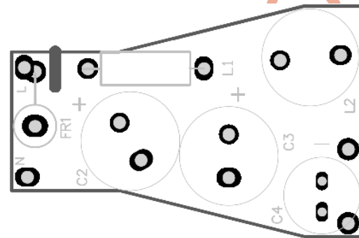
Top Layer
