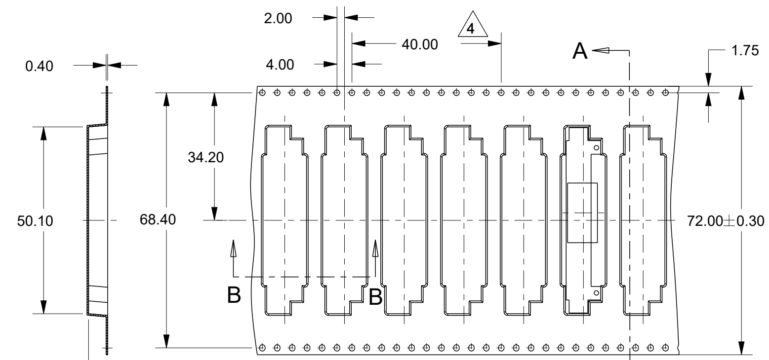
SECTION A-A
