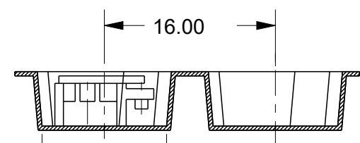
SECTION B-B SCALE 2:1
