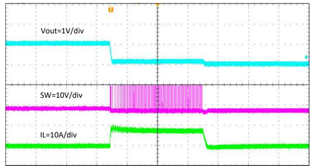
80us/div
