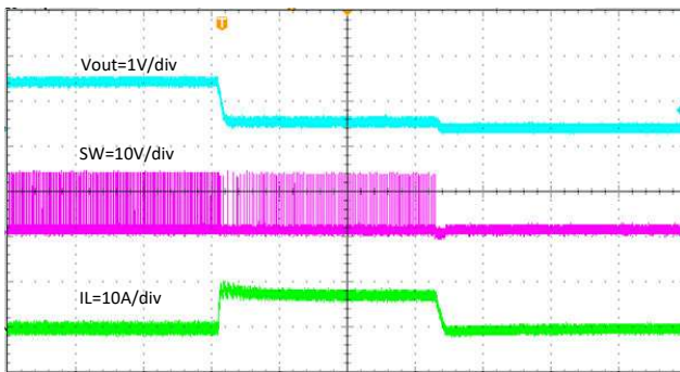
80us/div
