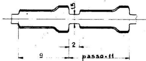
SEZ. A-A
