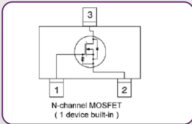
IXDN5 Schematica
