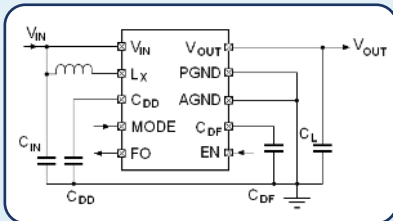
IXD2135 schematic
