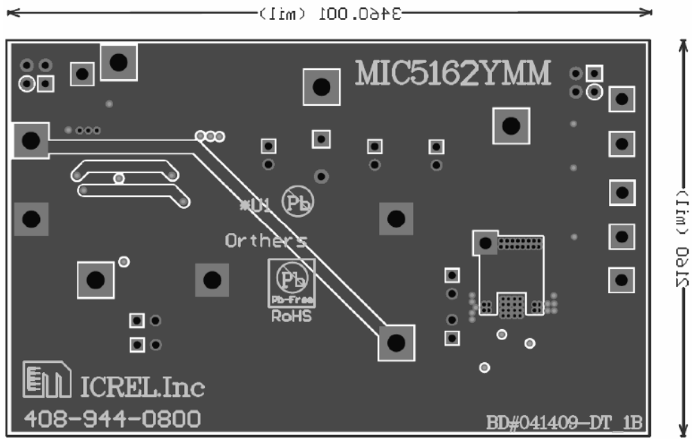
Bottom Layer
