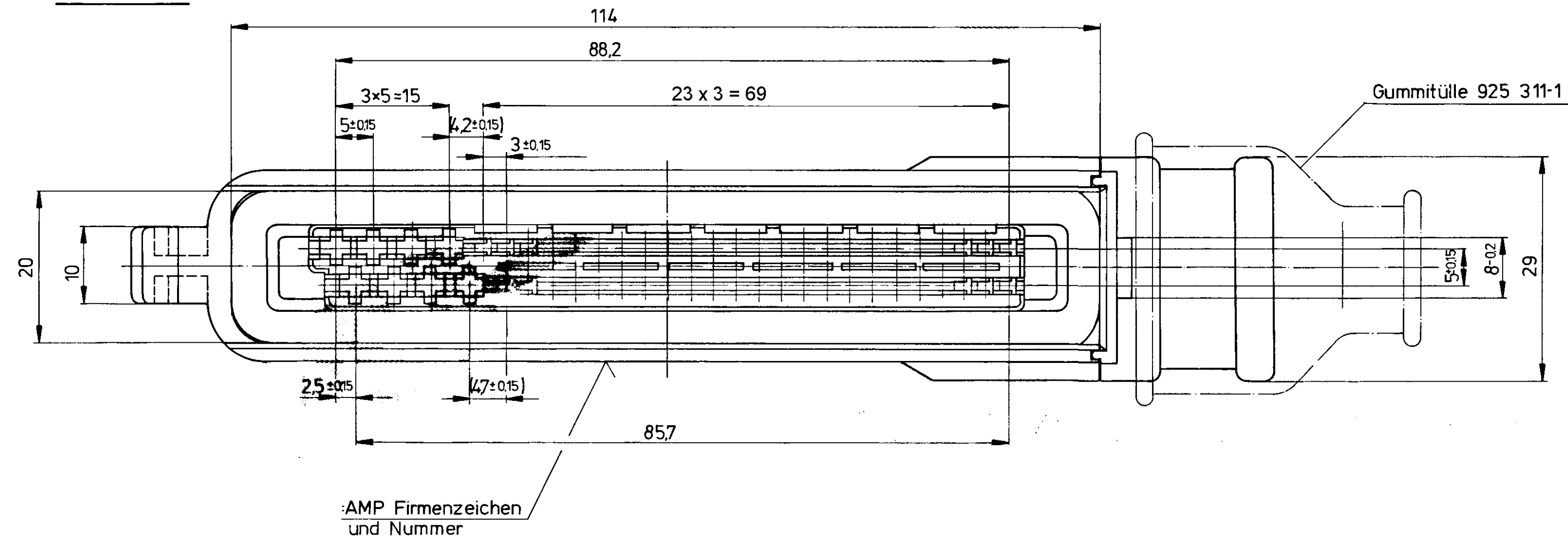
Ansicht X
