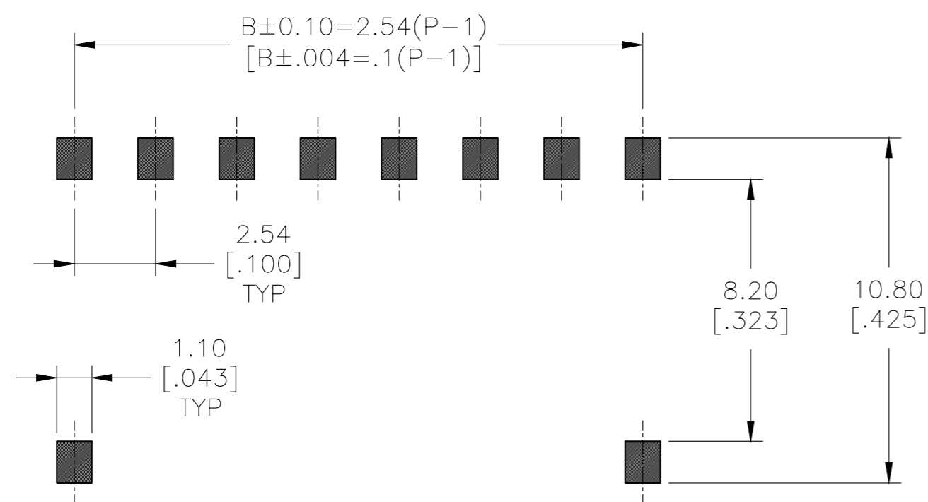
P.C.B. LAYOUT
