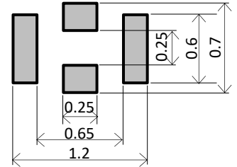
NFM18CC/18PC* *Except for NFM18PC106.
