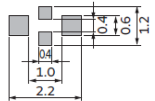
NFM18CC/18PC* *Except for NFM18PC106.
