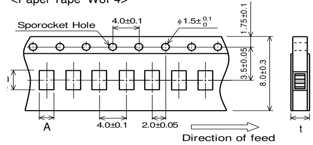
<Paper Tape W8P4>
