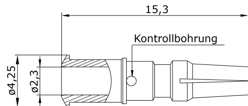
Hauptabmessungen Kontaktbuchse
