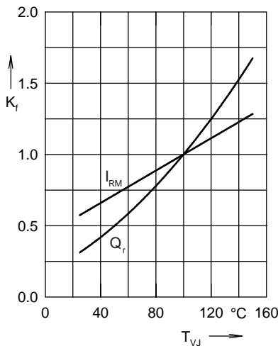
Fig. 21. Dynamic parameters Q_r , I_{RM} versus T_{VJ}
