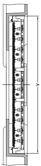
SECT. A-A (SCALE 2:1)
