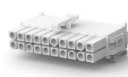
TE Part # 794210-1 20P MINI UMNL2 PLUG HSG UL94V0
