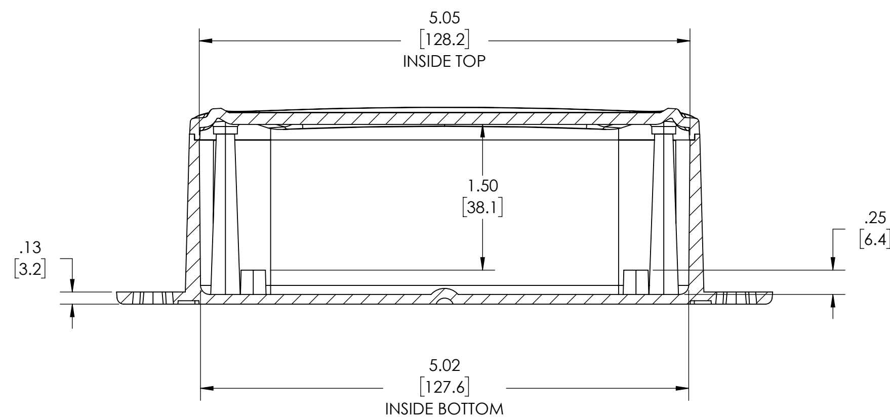
SECTION A-A
