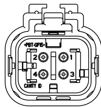
776524-4 SCALE 2:1
