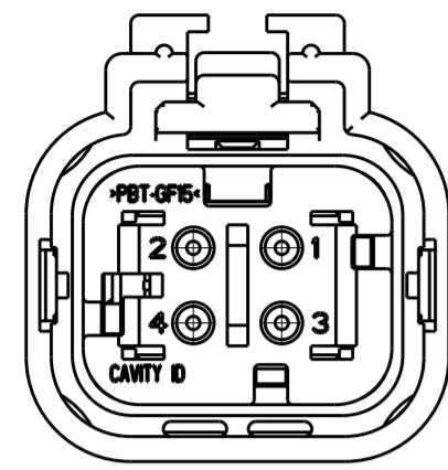
776524-2 SCALE 2:1
