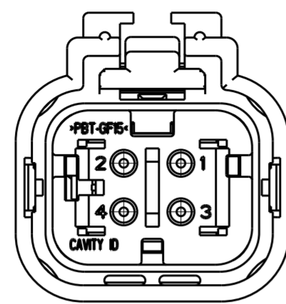
776524-3 SCALE 2:1
