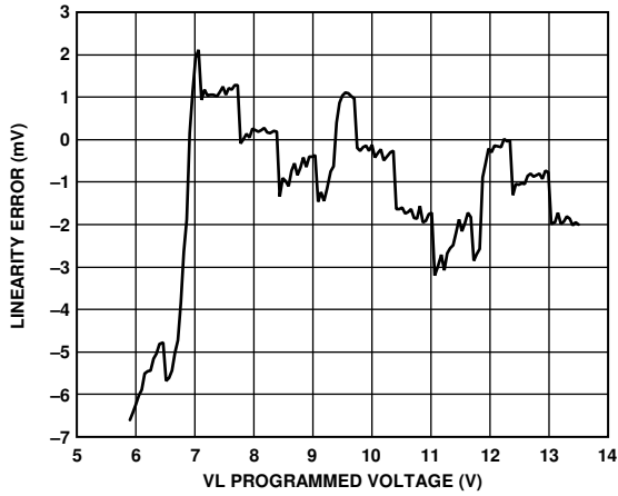
Figure 27. HVOUT VHH Linearity Error
