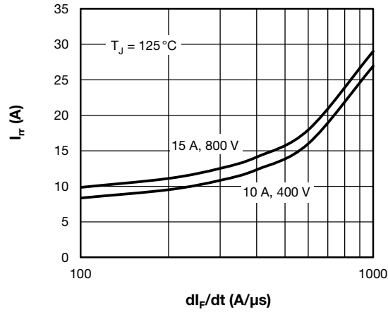
Fig. 9 - Typical Reverse Current vs. di F /dt, Per Leg
