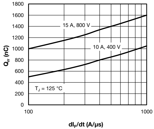
Fig. 8 - Typical Stored Charge vs. di F /dt, Per Leg
