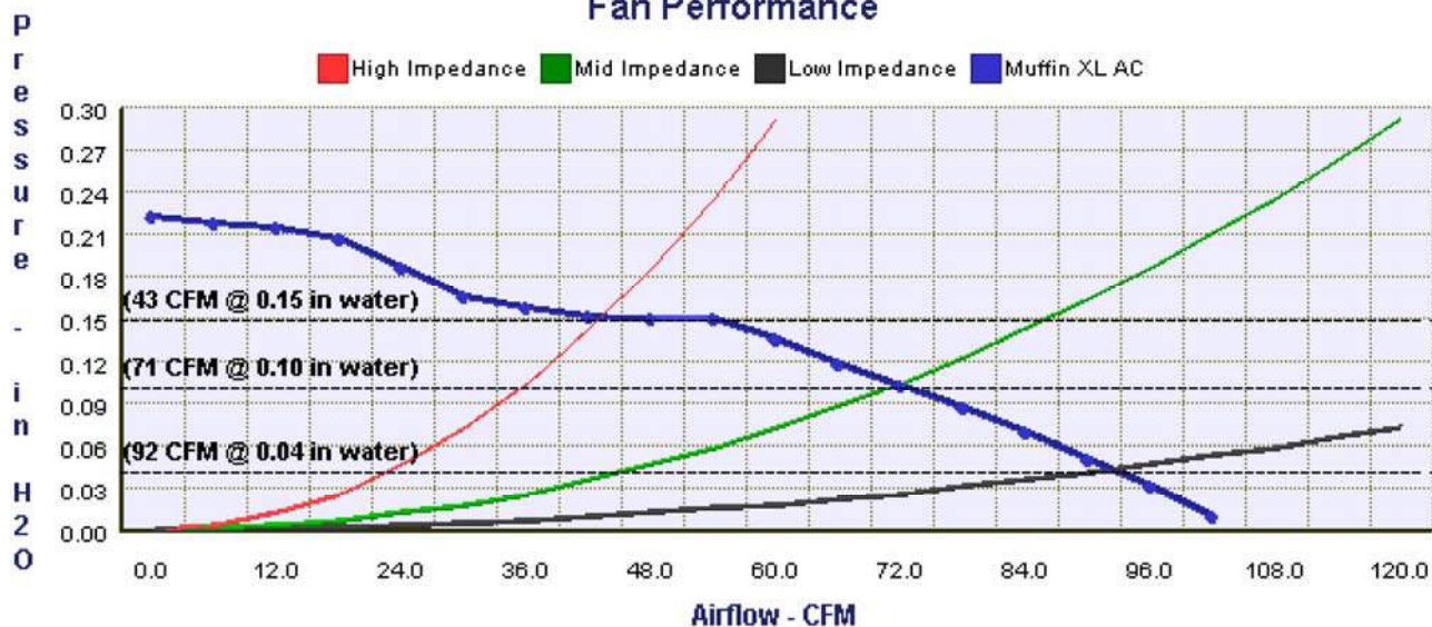
Fan Performance
