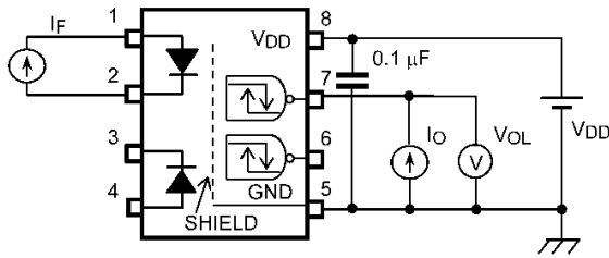
Fig. 12.1.1 VOL Test Circuit
