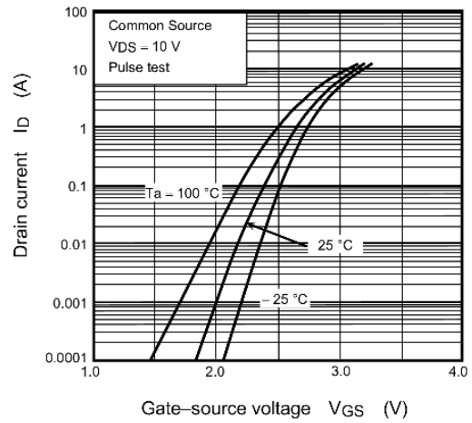
Fig. 7.2 I_D - V_{GS}
