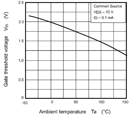
Fig. 7.6 V_{th} - T_a
