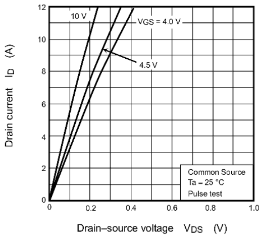
Fig. 7.1 I_D - V_{DS}
