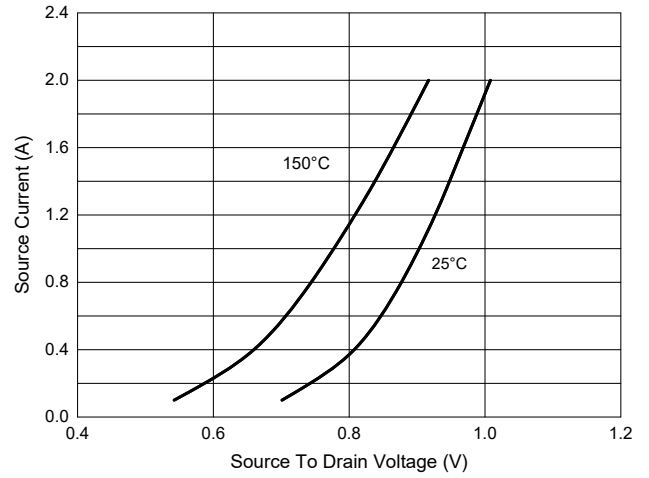
Fig. 8 - I_S - V_{SD}
