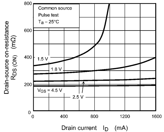
Fig. 7.1.4 R_{DS(ON)} - I_D
