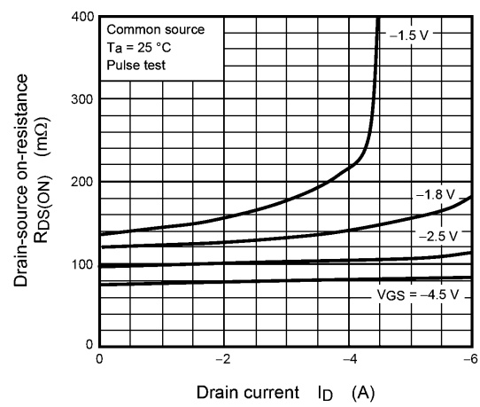
Fig. 8.4 R_{DS(ON)} - I_D
