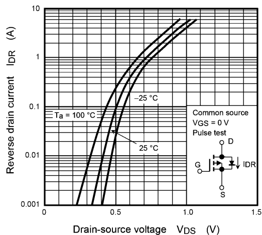
Fig. 8.8 I_{DR} - V_{DS}
