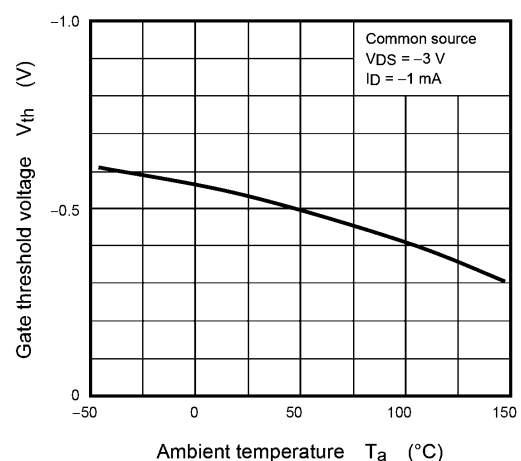
Fig. 8.6 V_{th} - T_a
