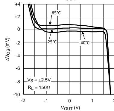
ΔV_Os vs. V_OUT
