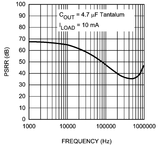
V_{BIAS} PSRR
