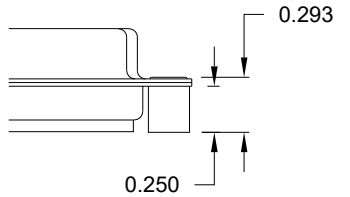
"02" // PCB SIDE
