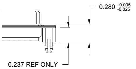
"90" // PCB SIDE **
