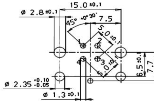
Leiterplattenbohrbild K-Seite
