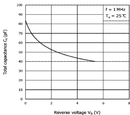
Fig. 9.3 C_t - V_R
