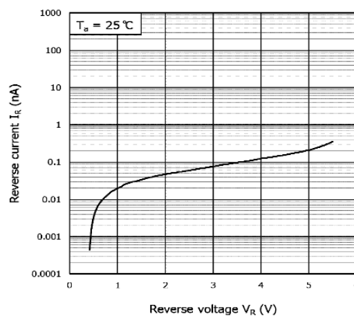
Fig. 9.2 I_R - V_R
