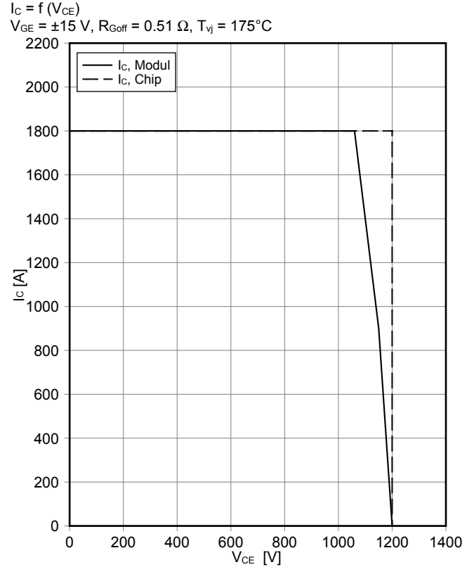
Sicherer Rückwärts-Arbeitsbereich IGBT, Wechselrichter (RBSOA) reverse bias safe operating area IGBT, Inverter (RBSOA) I_C = f(V_{CE}) V_{GE} = \pm 15\text{ V} , R_{Goff} = 0.51\ \Omega , T_{vj} = 175^\circ\text{C}
