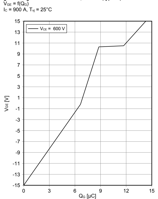
Gateladungs Charakteristik IGBT, Wechselrichter (typisch) gate charge characteristic IGBT, Inverter (typical) V_{GE} = f(Q_G) I_C = 900\text{ A} , T_{vj} = 25^\circ\text{C}
