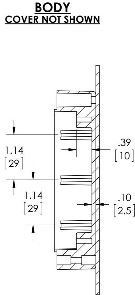
SECTION A-A
