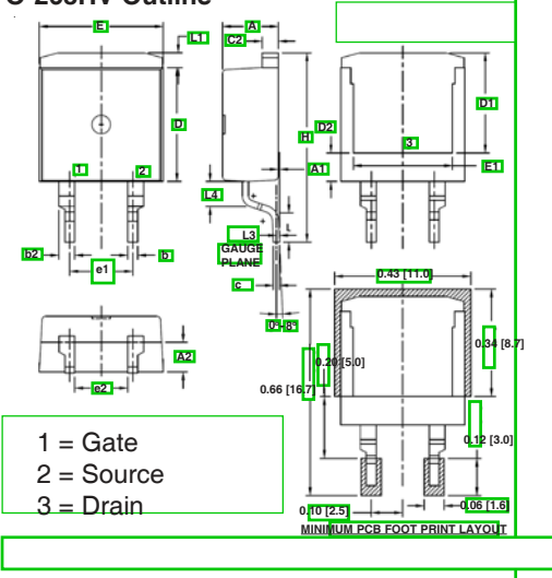
TO-263HV Outline
