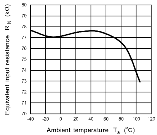
Fig. 12.10 R_{IN} - T_a
