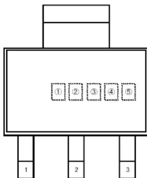
SOT-223
