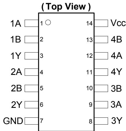
SO-14 / TSSOP-14
