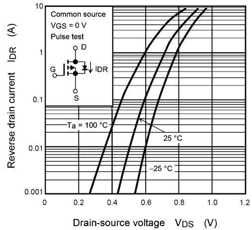
Fig. 8.8 I_{DR} - V_{DS}
