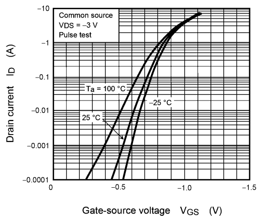
Fig. 8.2 I_D - V_{GS}
