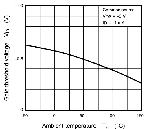
Fig. 8.6 V_{th} - T_a
