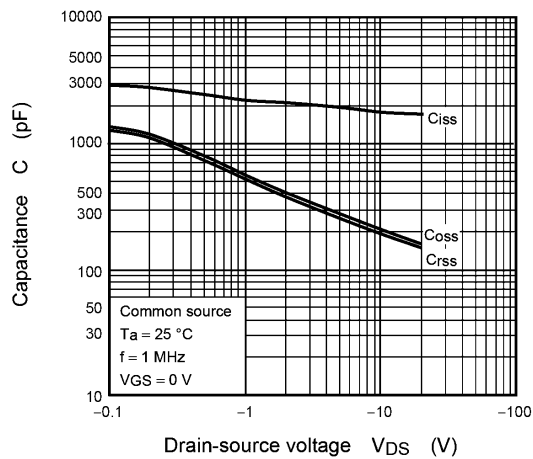
Fig. 8.9 C - V_{DS}
