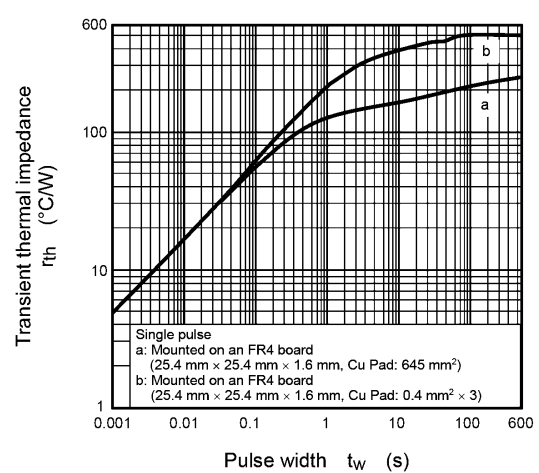
Fig. 8.12 r_{th} - t_w
