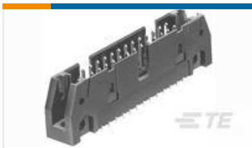
TE Part # 3-1761679-1 IDC LOW PRO HDR 34P VERT BLUE
