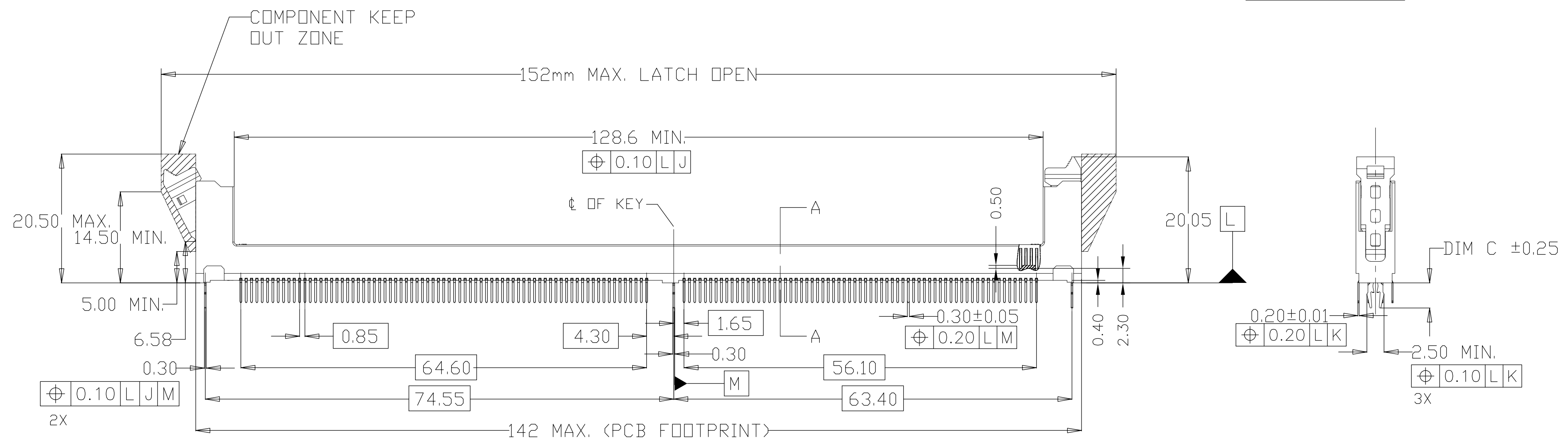
SECTION A-A
