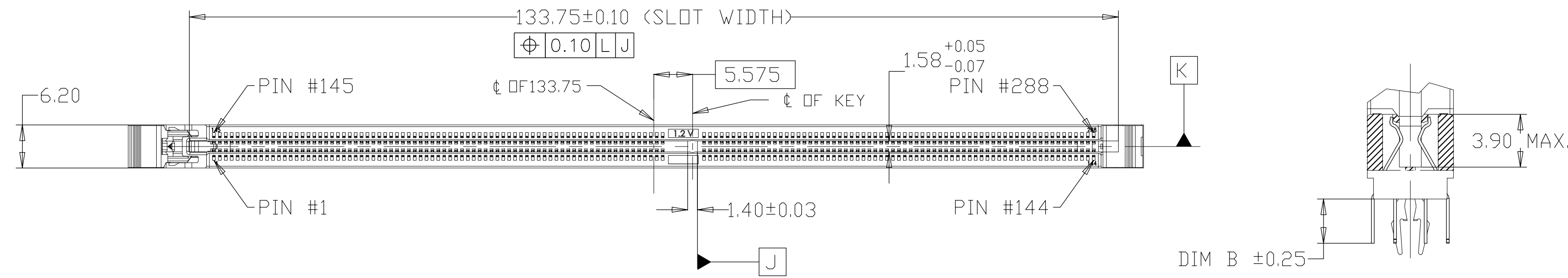
SECTION A-A
