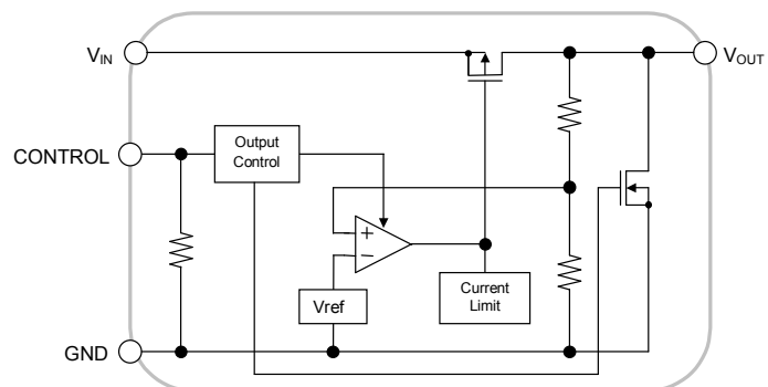
NJU7744
