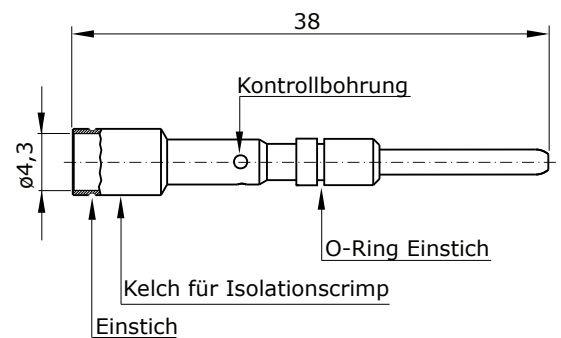
Hauptabmessungen Kontaktstift
