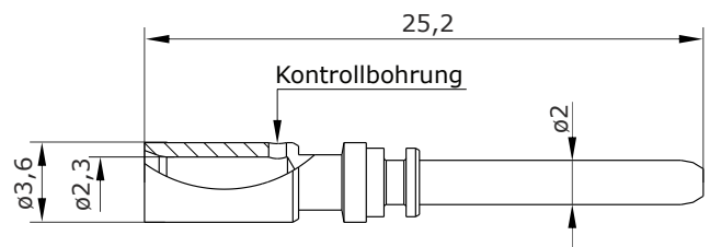
Hauptabmessungen Kontaktstift
