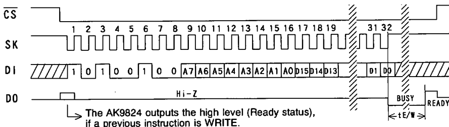
WRITE (AK9824)
