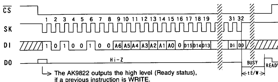
WRITE (AK9822)
