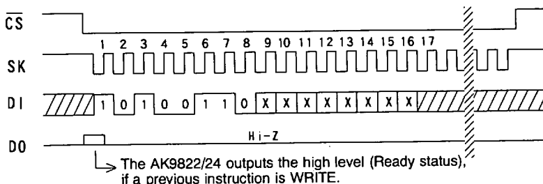
PDDS (AK9822/24)
