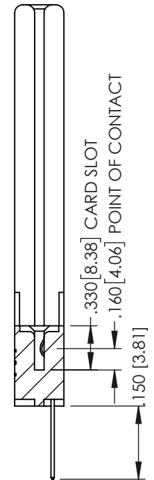
SECTION A-A
