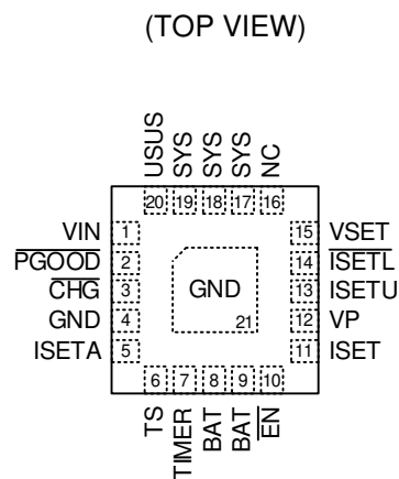
WQFN-20L 3x3
