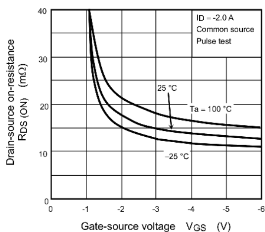
Fig. 7.4 R_{DS(ON)} - V_{GS}
