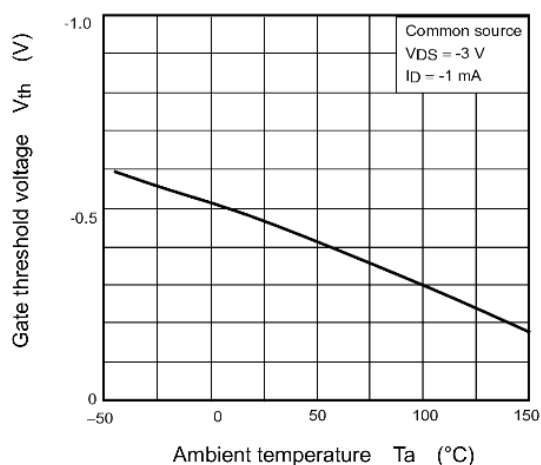
Fig. 7.7 V_{th} - T_a
