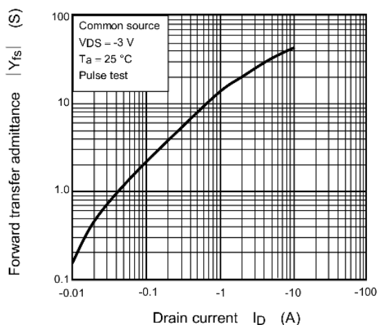
Fig. 7.8 |Y_{fs}| - I_D
