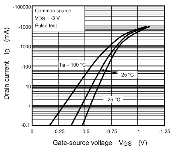
Fig. 7.2 I_D - V_{GS}
