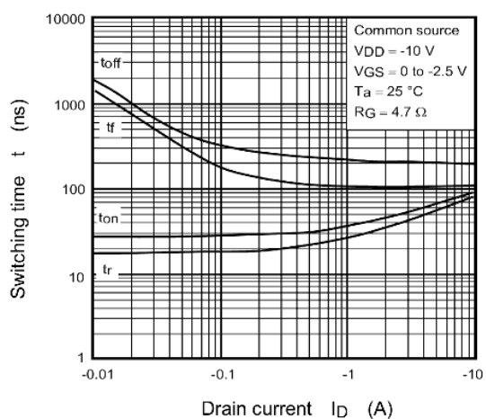
Fig. 7.11 t - I_D
