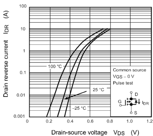
Fig. 7.9 I_{DR} - V_{DS}
