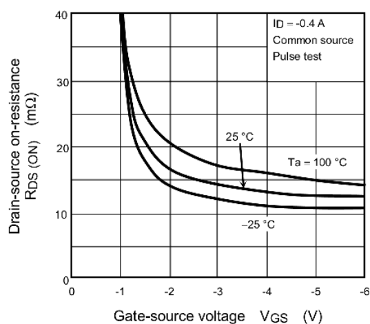
Fig. 7.3 R_{DS(ON)} - V_{GS}
