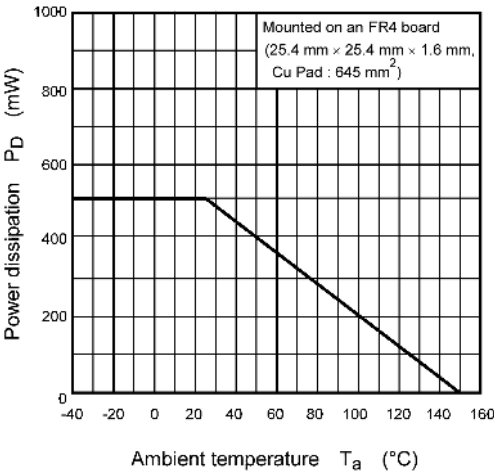
Fig. 7.14 P_D - T_a
