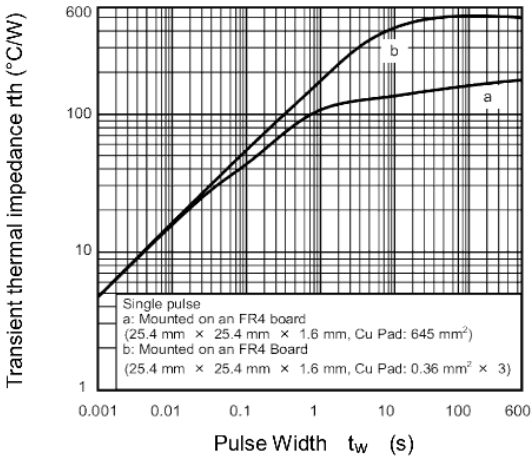
Fig. 7.13 r_{th} - t_w
