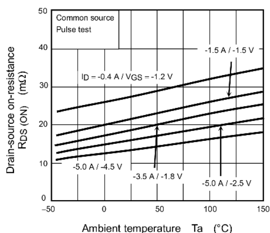
Fig. 7.6 R_{DS(ON)} - T_a
