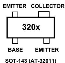
SOT-143 (AT-32011)
