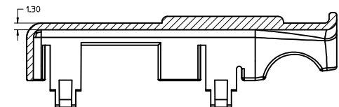
SECTION A-A SCALE 3:1
