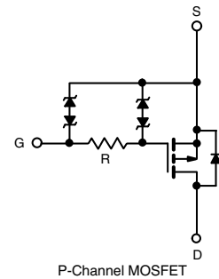
P-Channel MOSFET
