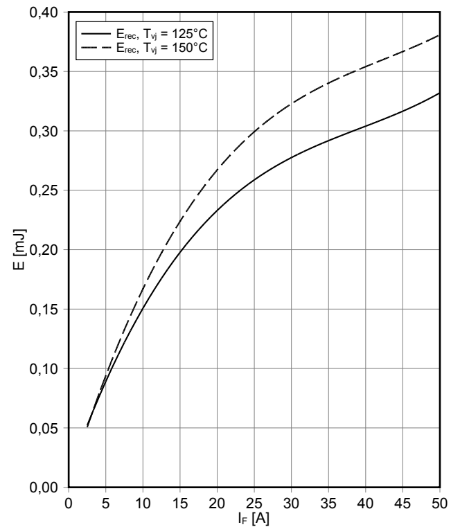
Schaltverluste Diode, D2 / D3 (typisch) switching losses Diode, D2 / D3 (typical) E_{rec} = f(I_F)
